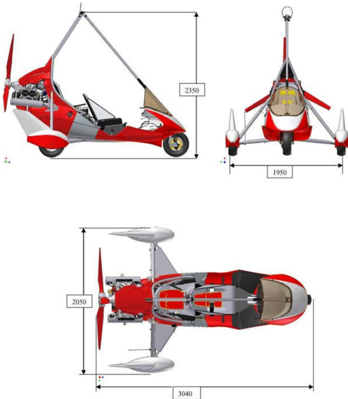
Figure 3-1 : Tanarg 912 - 3 Vues
