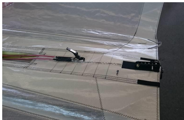
Figure 5-2 : Cheminement des câbles d'étarquage
